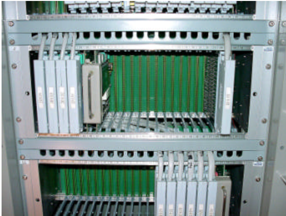
Alte Netzleitunterstation von Landis und Gyr vor Umbau
